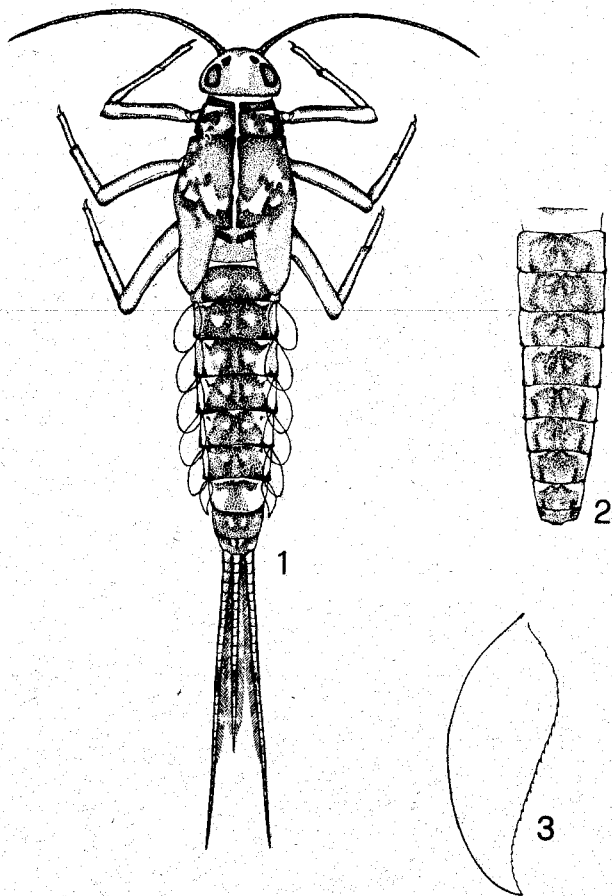
Figg. 1-3 Baetis digitatus Bengtsson: ninfa (1); urotergiti di un altro individuo (2); tracheobranchia del VII urite (3).
