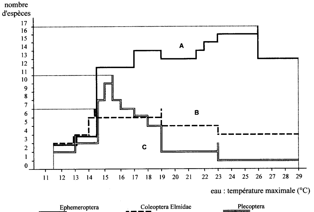
Fig. 1. Nombres d'espèces d'Ephémères (A), de Coléoptères Elmidae (B) et de Plécoptères (C) en fonction de la température maximale de l'eau.
