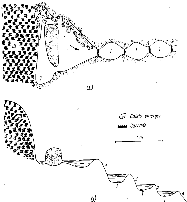
Fig. 1. Plan d'un secteur du petit affluent de la Roztoka. Pod Mostem: a) vue d'en haut, b) coupe longitudinale.
