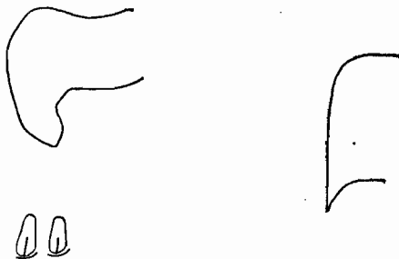
Obr. 1. Tvar pronota.
