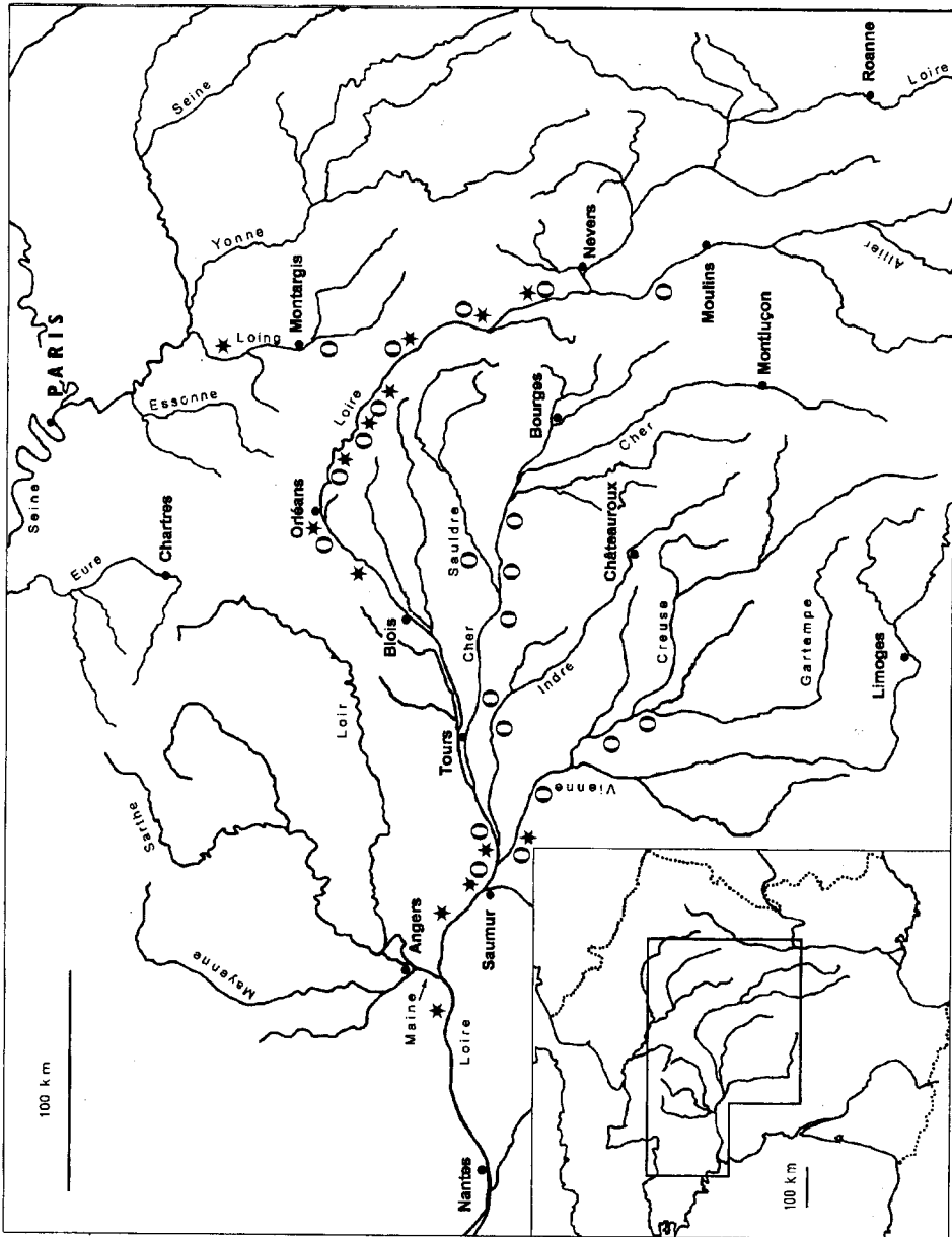
Carte 1. Zone géographique prospectée (les astérisques indiquent les sites à Cercobranchys minutus , les cercles vides ceux à Brachycercus europaeus ).
