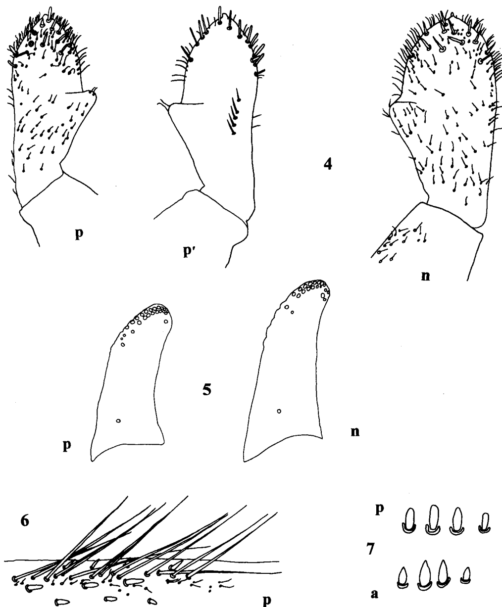
Pl. 2. Structures larvaires (au dernier stade) de Baetis spp. (p : pasquetorum n. sp.; a : alpinus ; n : nubecularis ) [même échelle]. 4 : palpe labial (p, n : face ventrale; p' : face dorsale). 5 : paraglosse. 6 : bord postérieur du fémur I. 7 p, a : écailles dorsales de la partie proximale des fémurs.
