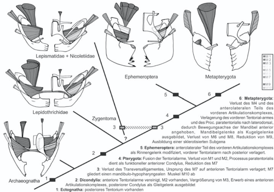
Abb. 1: Phylogenetisches Argumentationsschema der basalen Aufspaltungseignisse im Stammbaum der Ectognatha, impliziert durch den Bau der Mandibel (verändert nach Staniczek 2001).
