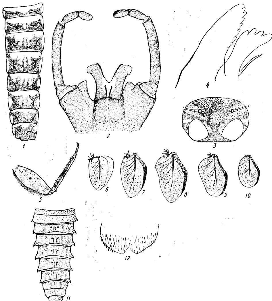
Рис. 1. Детали строения имаго и личинки E. rubeus : 1 — расправленные I—X тергиты брюшка самца имаго; 2 — гениталии самца; 3 — голова; 4 — зубы левой мандибулы; 5 — передняя нога; 6—8 — жабры I—III пары; 9—10 — жабры VI—VII пары; 11 — I—X тергиты брюшка личинки; 12 — посгенитальная пластинка.
