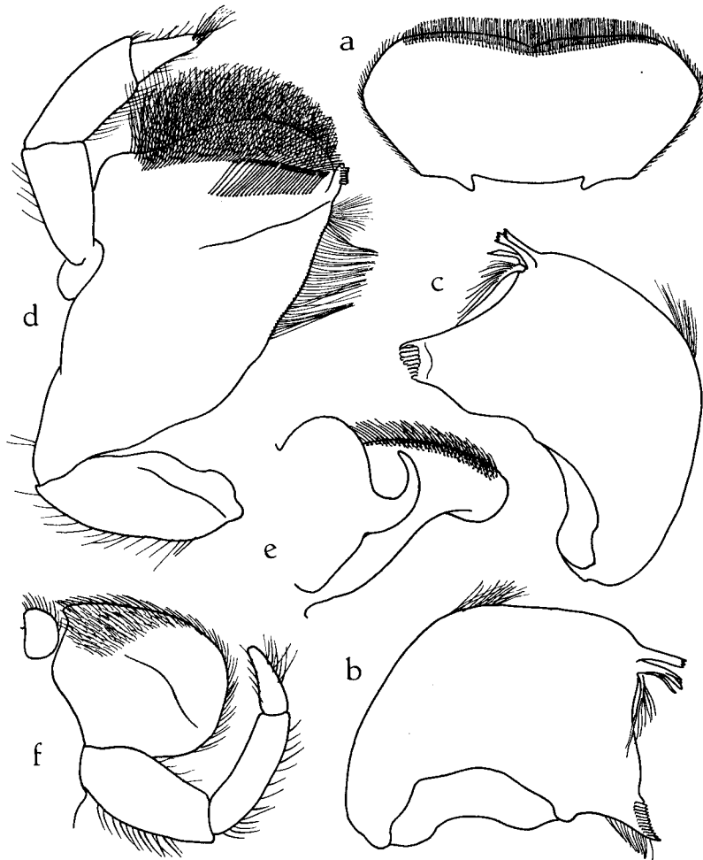
Fig. 2. — Atalophlebioides inequalis sp. nov., larve holotype, pièces buccales (vue ventrale, sauf le labre); \times 50 .
