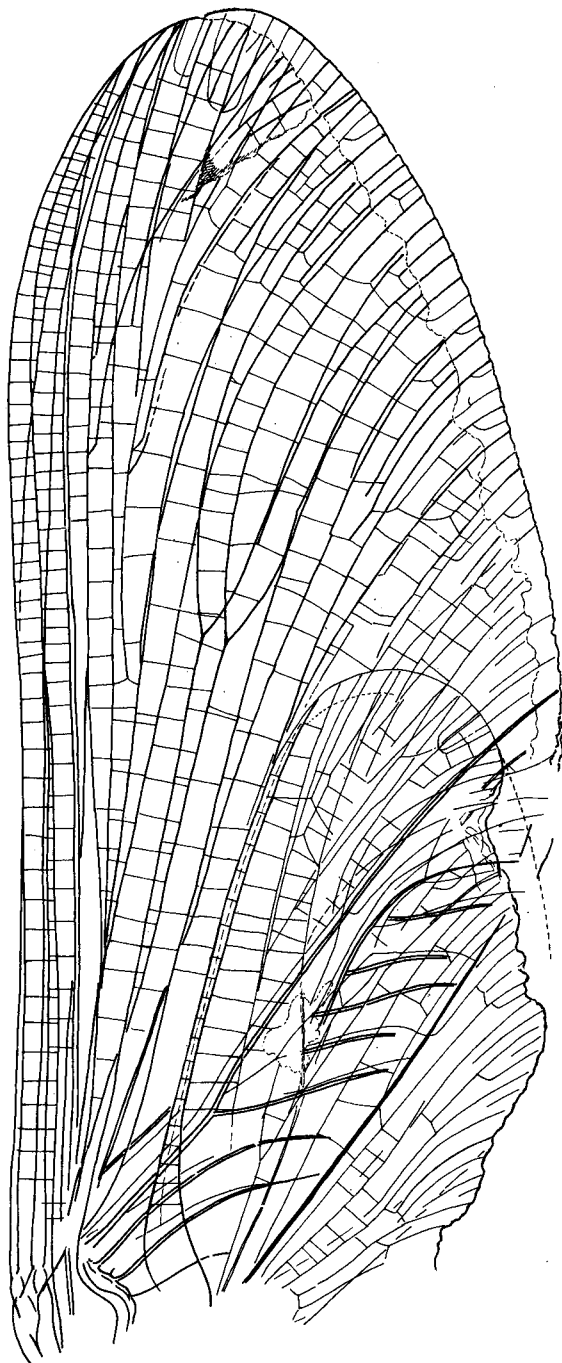
Fig. 1. — Hexagenites cellulosus (HAGEN) ♀ (Holotype de Paedephemera multinervosa (OPPENHEIM) in Bayer. Staatssamml. Pal. & hist. Geol., München). Les quatre ailes superposées, en vue latérale gauche; \times 8 env. On notera que la superposition des ailes ne facilite pas l'identification des nervures et leur attribution à l'une ou l'autre aile; la longueur exacte (et par conséquent les attaches) des nervures transverses ne peut toujours être garantie.
