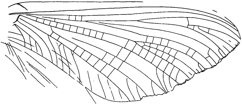
Fig. 2. — Oligisca schwertschlageri (HANDLIRSCH), Holotype, aile antérieure droite; × 7 env. (Phil.-Theol. Hochschule, Eichstätt).
