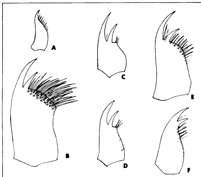
FIGURE 1. Isoperla . Lacinia of: A - I. nana ; B - I. lata ; C - I. cotta ; D - I. richardsoni ; E - I. marlynia ; F - I. signata .
