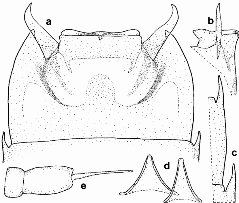
Abb. 4. Caenis basuto ; Männchen. - a. Genitalia; - b. Lateralansicht von a; - c. Lateralfortsätze von Segment 6 und 7; - d. Prosternaldreieck; - e. Fühler: Pedicellus und Basis der Geißel.
